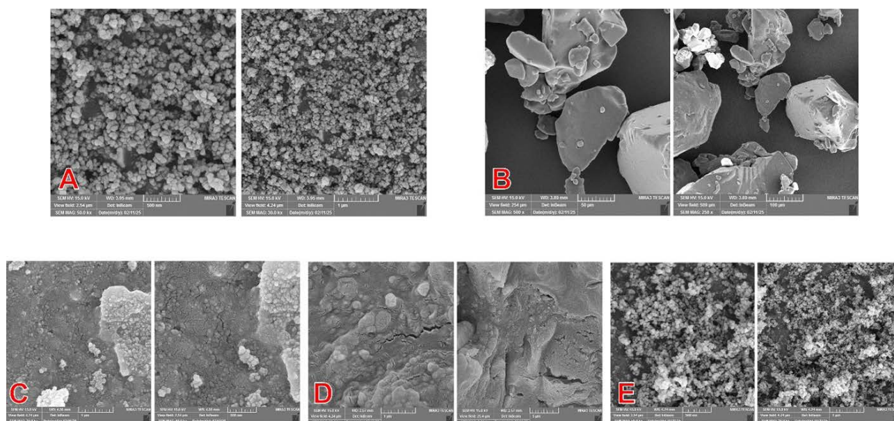
Figure 3. Representative FESEM images: A) \text{TiO}_2 . B) PLGA. C) PLGA+ \text{TiO}_2 (PVP), D) PLGA+ \text{TiO}_2 (without PVP). E) PLGA+ \text{TiO}_2 (physical mix)
